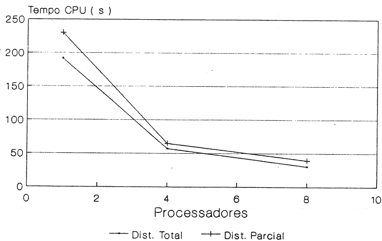
Figura 5 - Tempos de resposta junção de 100x1000 tuplas
