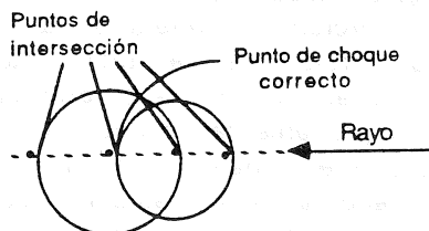
Fig 4. Intersección rayo-superficies
