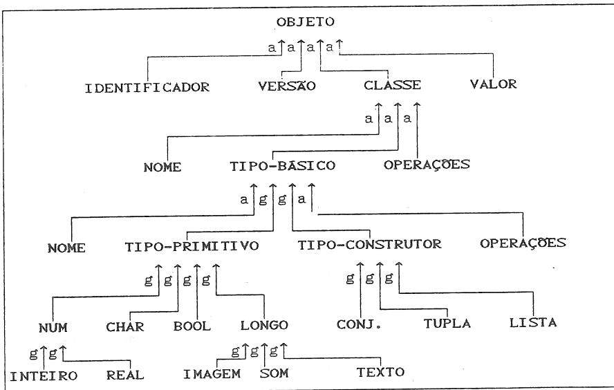
FIGURA 1: Representação gráfica de um objeto no MORSO.
